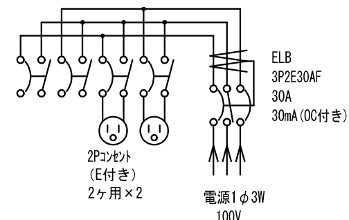
結線図
